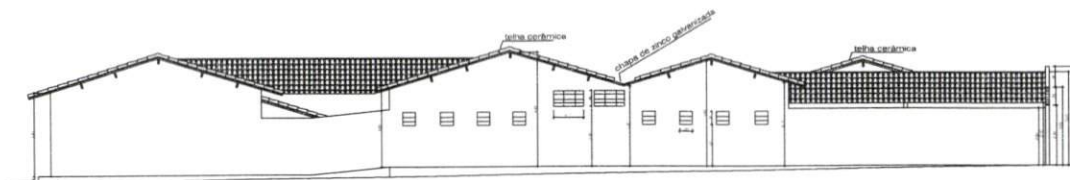
FAXADA LATERAL
